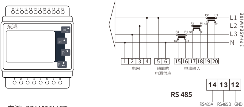
图7.3 东鸿三相电表
