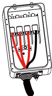
图5.9交流电缆已连接到端子
