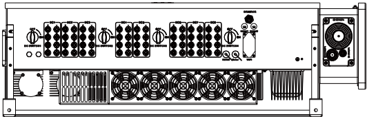
图1.2 底视图
