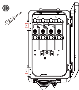
图5.7交流接线盒
