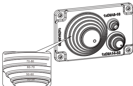
图5.8密封圈
