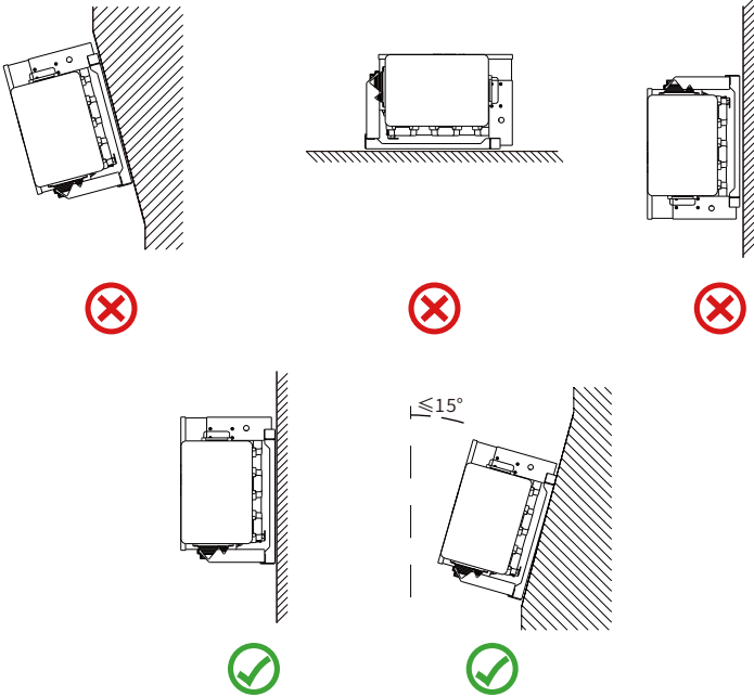
图4.2 安装角度
