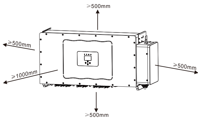
图4.3 安装间隙
