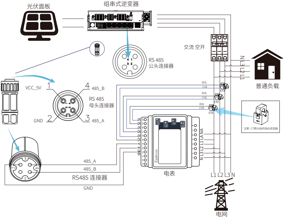
图7.4 东鸿三相电表连接
