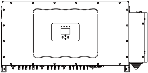
图1.1 前视图
