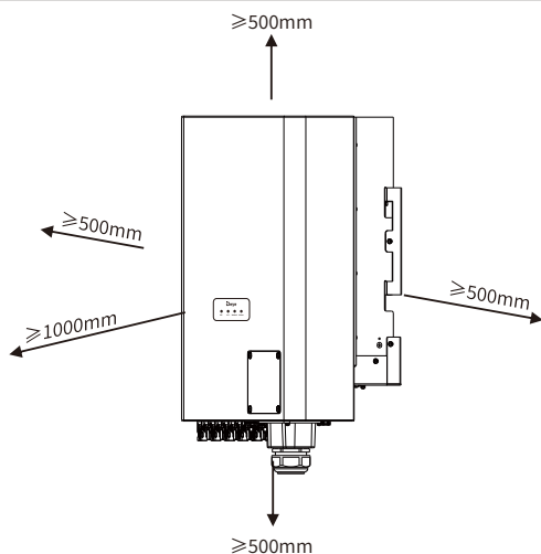
图4.3 安装间隙
