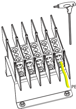
图5.8 外壳接地线的安装
