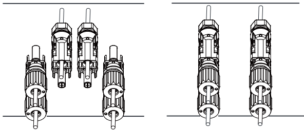
图5.6 直流输入端连接
