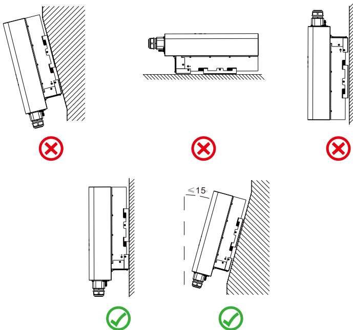
图4.2 安装角度
