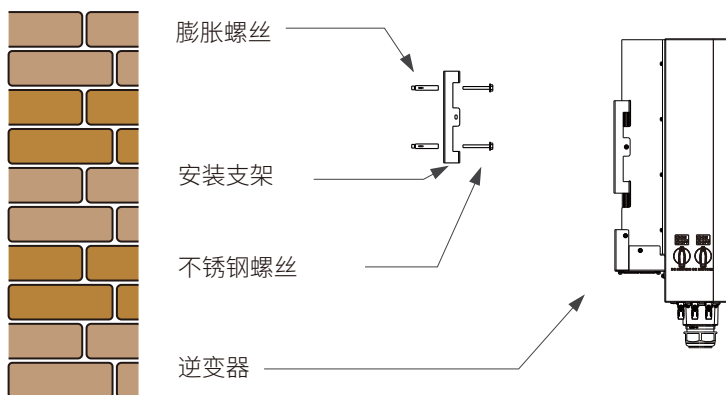
图4.4 逆变器的安装
