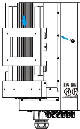
图4.6 逆变器的安装
