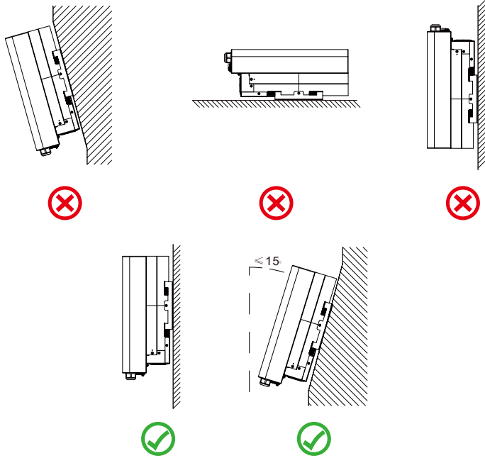
图4.2 安装角度
