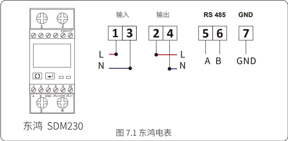
东鸿电表的系统连接图
