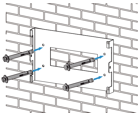
图4.5 逆变器支架的安装
