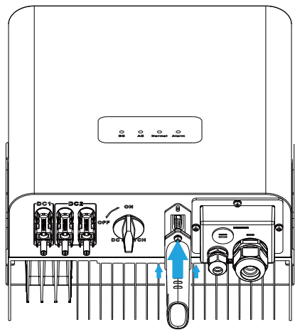
图5.13 数据采集器安装图示
