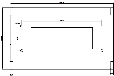
图4.5 逆变器支架的安装
