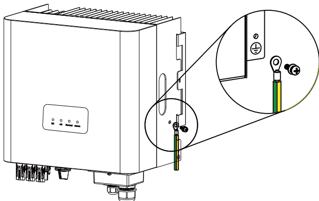
图5.11 外壳接地线的安装
