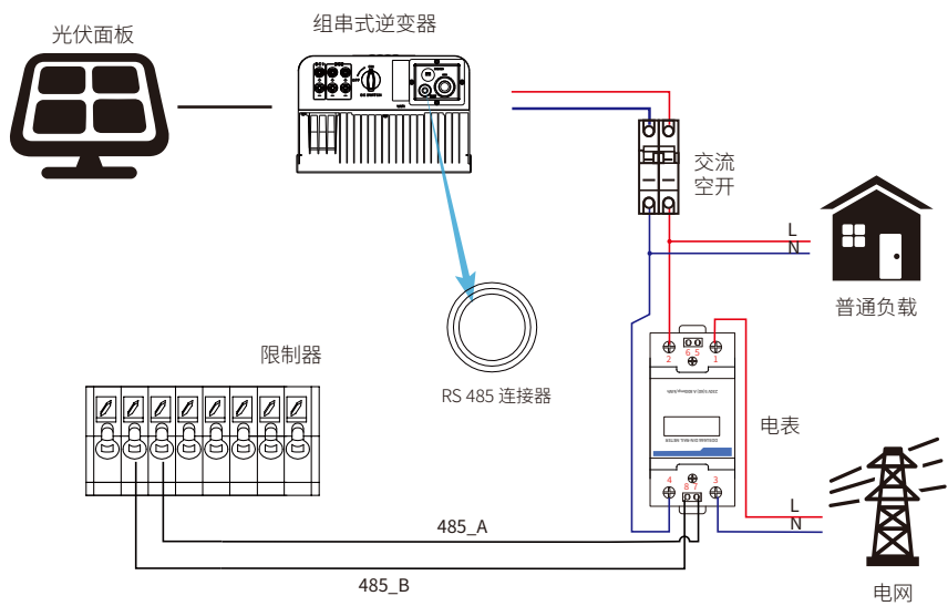
图 7.4 正泰单相电表连接
