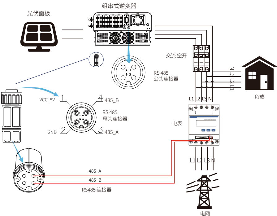
图7.6 正泰电表连接
