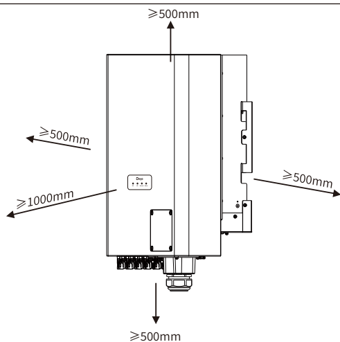
图4.3 安装间隙
