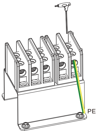
图5.8 外壳接地线的安装
