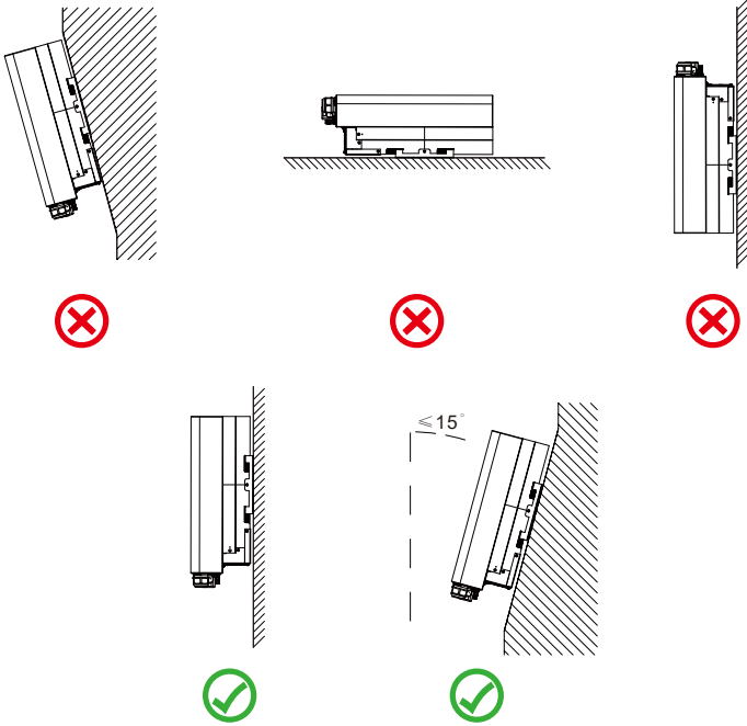
图4.2 安装角度
