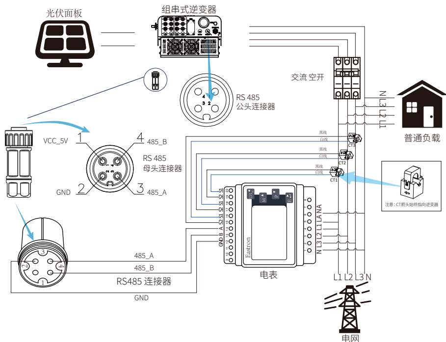
图6.4 东鸿三相电表连接
