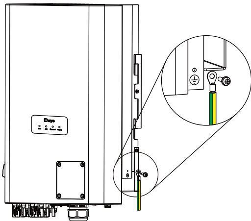
图5.8 外壳接地线的安装
