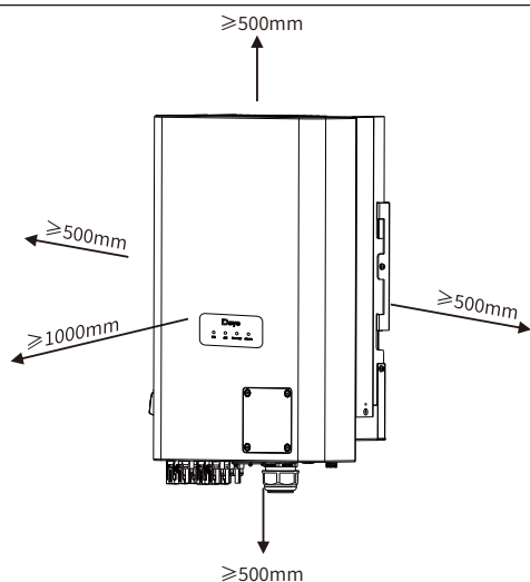
图4.3 安装间隙
