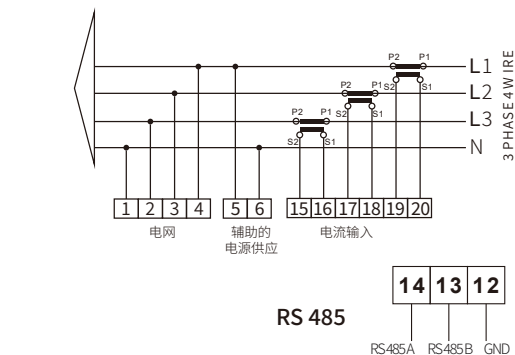
图6.3 东鸿三相电表
