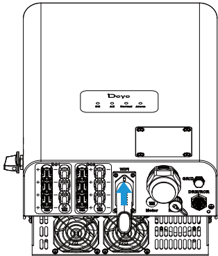
图5.10 数据记录仪安装图示
