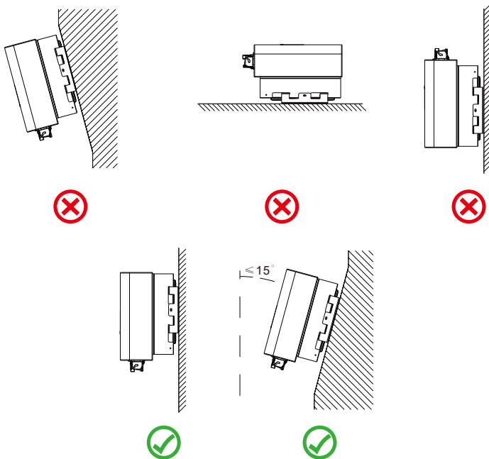
图4.2 安装角度
