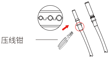
图5.4 将压接端子压接到电线上
