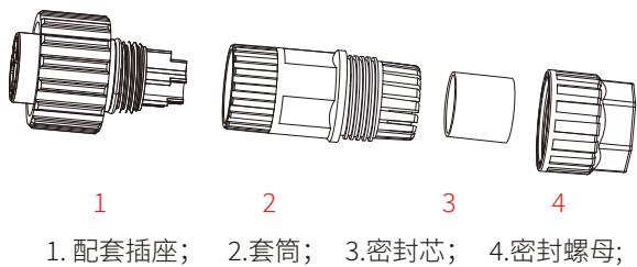
图5.7 交流连接器结构
