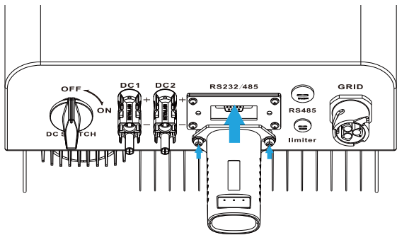
图5.13 数据采集器安装图示
