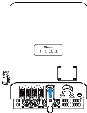
图5.10 数据记录仪安装图示
