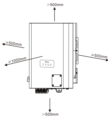
图4.3 安装间隙
