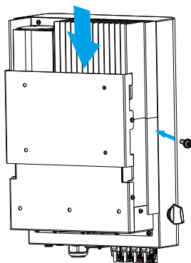
图4.6 逆变器的安装
