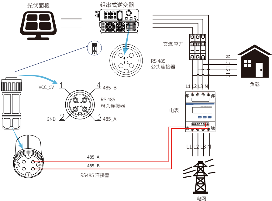
图6.6 正泰电表连接
