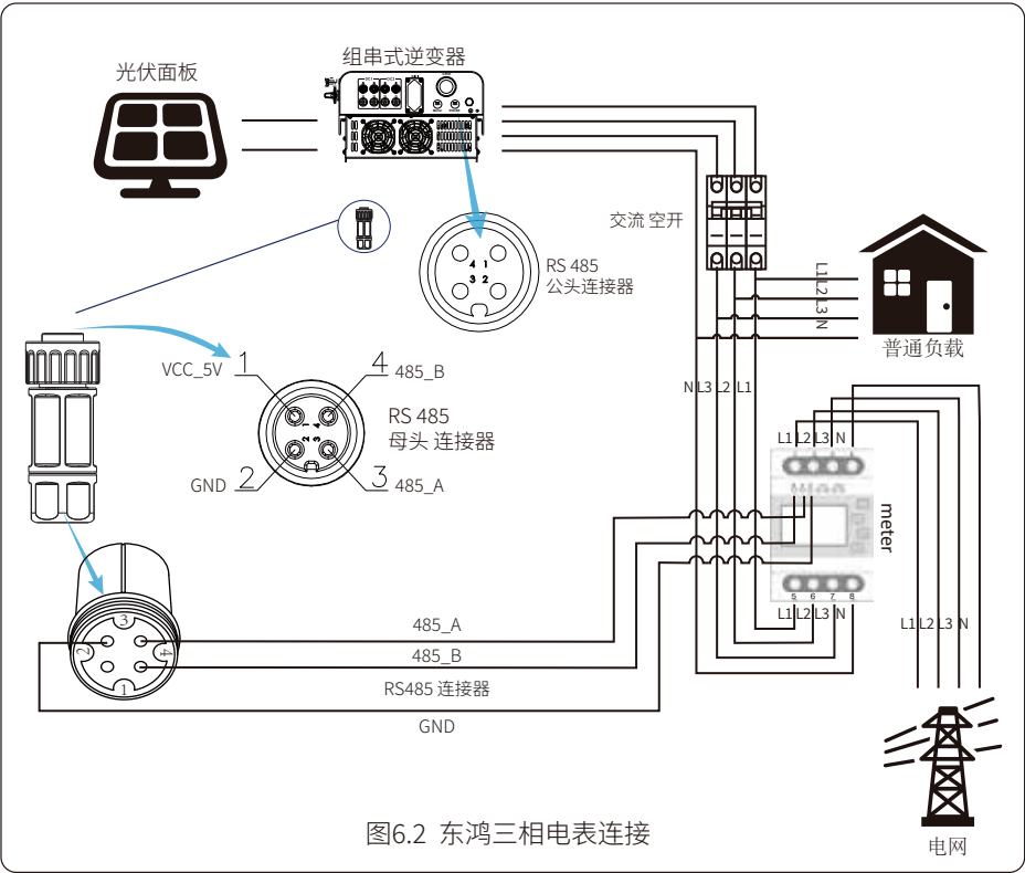
东鸿 SDM630-Modbus V2 图6.1 东鸿三相电表
