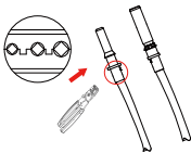
图5.4 将压接端子压接到电线上
