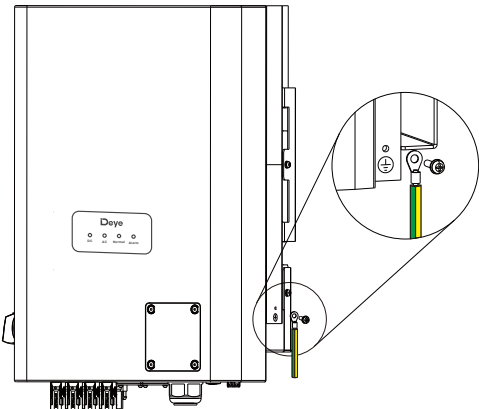
图5.8 外壳接地线的安装
