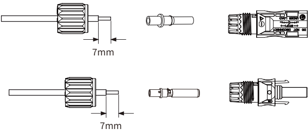
图5.3 拆卸连接器螺帽
