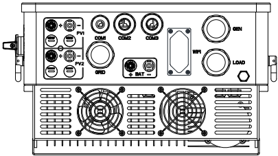
SUN-8/10K-SG01HP3-EU-AM2
