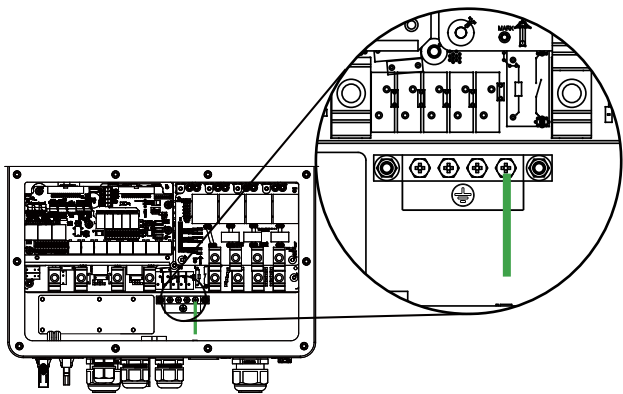
接地连接（铜线）（旁路）
