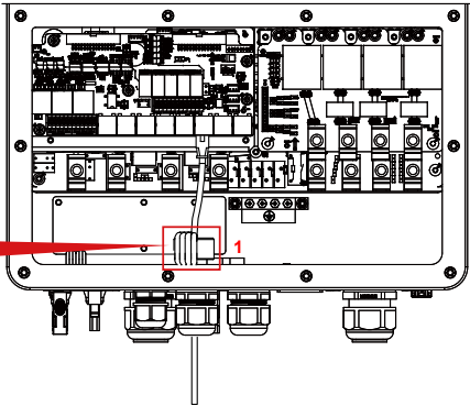
图3.6直流输入连接
