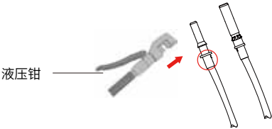
图3.4将接触引脚压接到导线上
