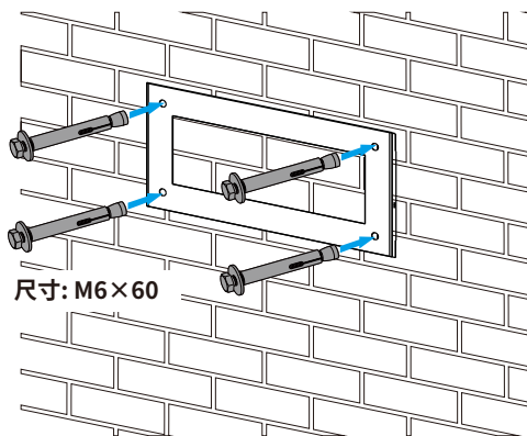
逆变器安装支架安装
