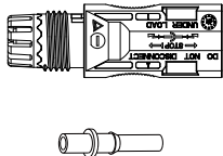
图3.2 DC-接口
