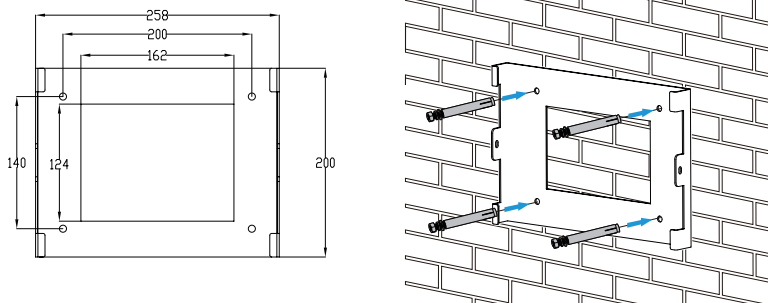
图4.5 逆变器支架的安装
