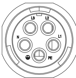
图5.9 交流连接器孔样式
