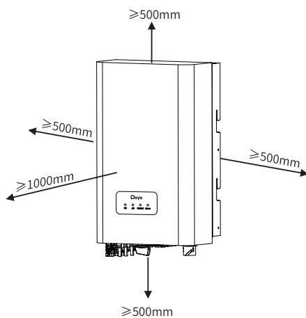
图4.3 安装间隙
