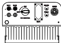
图1.2 底视图
