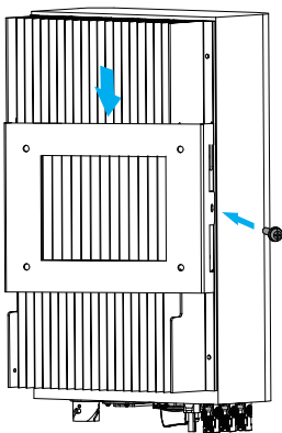
图4.6 逆变器的安装
