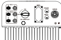
图1.4 底视图
