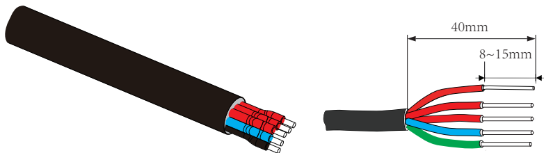
图5.8 剥除交流软线外层
