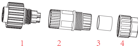
1. 配套插座； 2. 套筒； 3. 套筒； 4. 密封螺母
