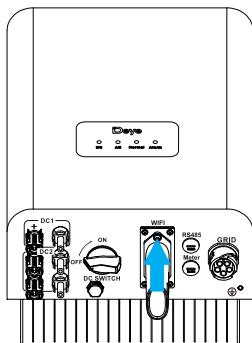
图5.13 数据记录仪安装图示
