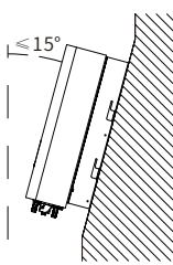
图4.2 安装角度
