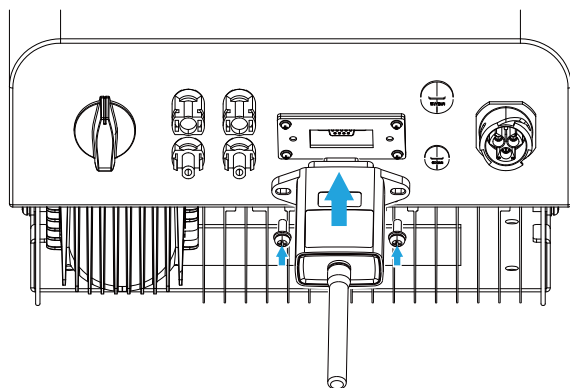
图5.13 数据采集器安装图示
