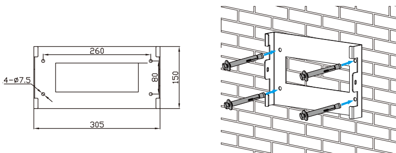
图4.5 逆变器支架的安装
