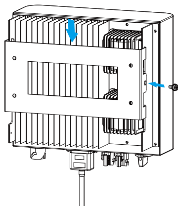
图4.6 逆变器的安装
