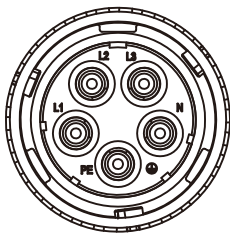
图5.9 交流连接器孔样式
