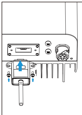
图5.13 数据记录仪安装图示
