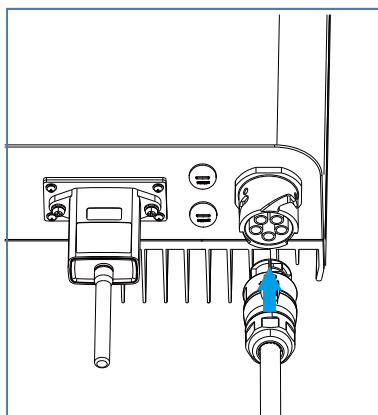
图5.10 交流输入的连接
