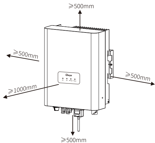
图4.3 安装间隙
